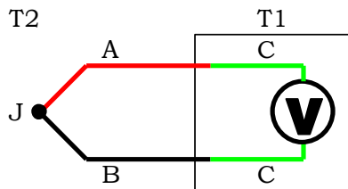
图 5.1 热电偶效应
